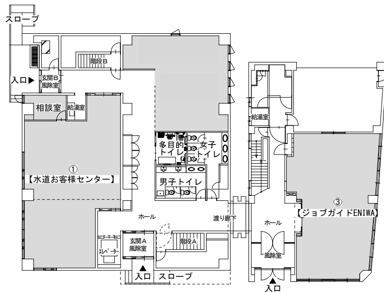
恵庭市第2庁舎 1階 平面図
