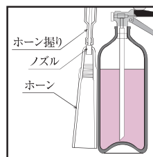
二酸化炭素消火器のホーン
