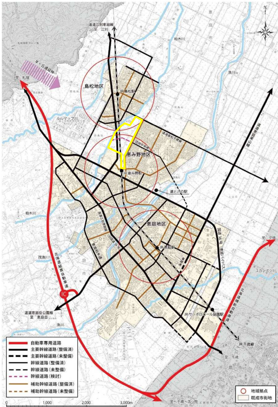
図 3-2 道路整備方針図
