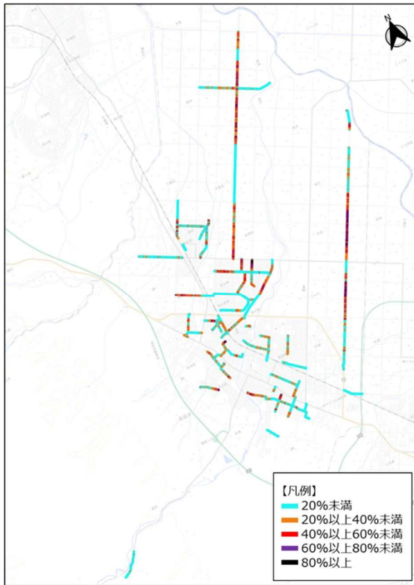
図 2-8 準幹線道路の調査結果（左：ひび割れ率、右：わだち掘れ量）
