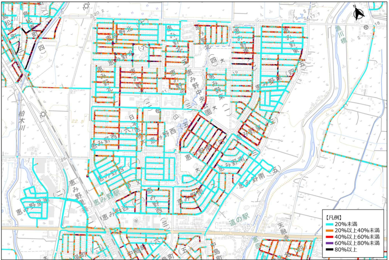
図 2-12 生活道路のひび割れ率調査結果（恵み野地区）
