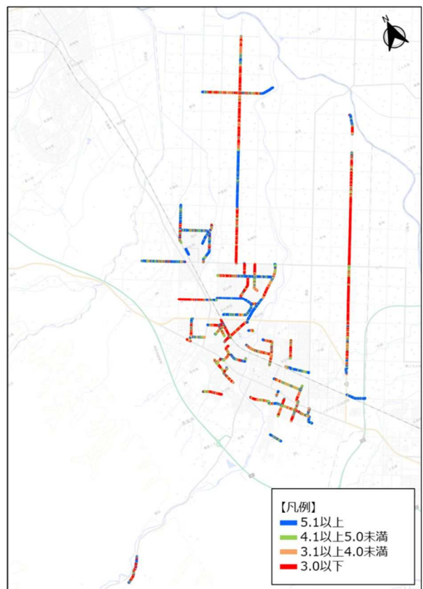
図 2-9 準幹線道路の調査結果（左：IRI、右：MCI）
