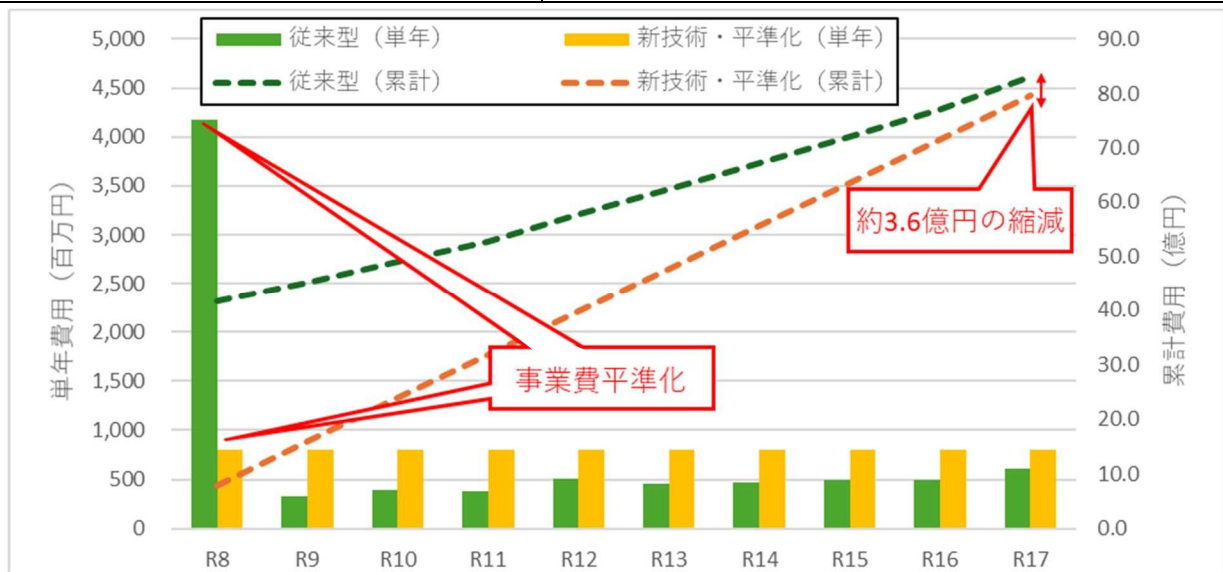
図 3-8 従来型と新技術・平準化型の LCC 縮減効果
