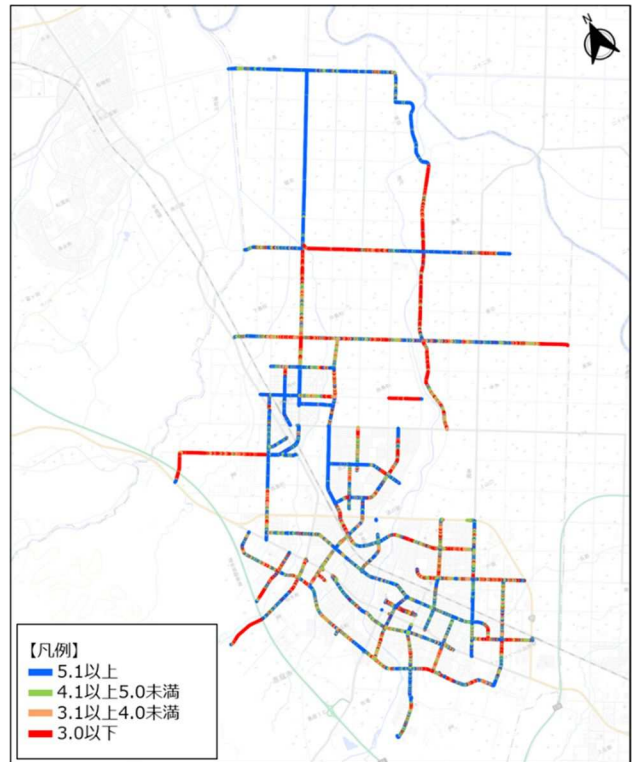
図 2-7 幹線道路の調査結果 (左：IRI、右：MCI)
