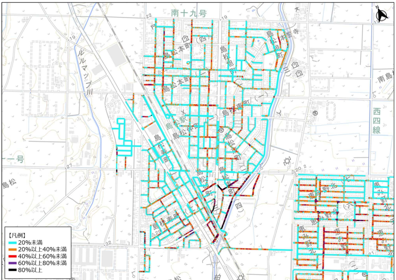
図 2-13 生活道路のひび割れ率調査結果（島松地区）
