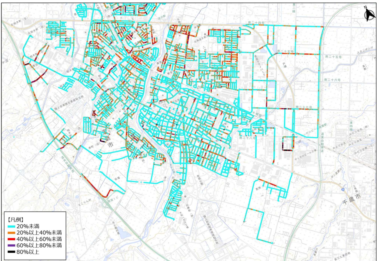
図 2-10 生活道路のひび割れ率調査結果
