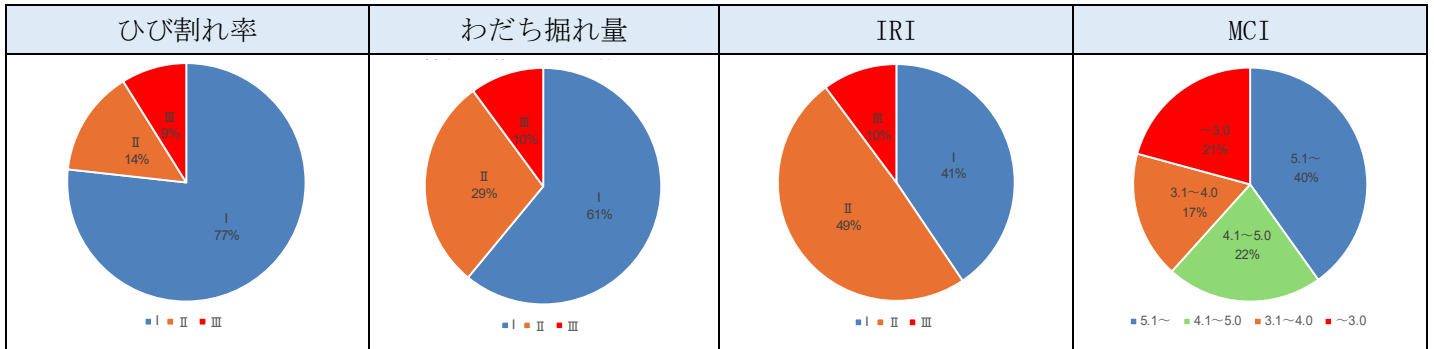
図 2-3 幹線道路の診断区分割合比較
