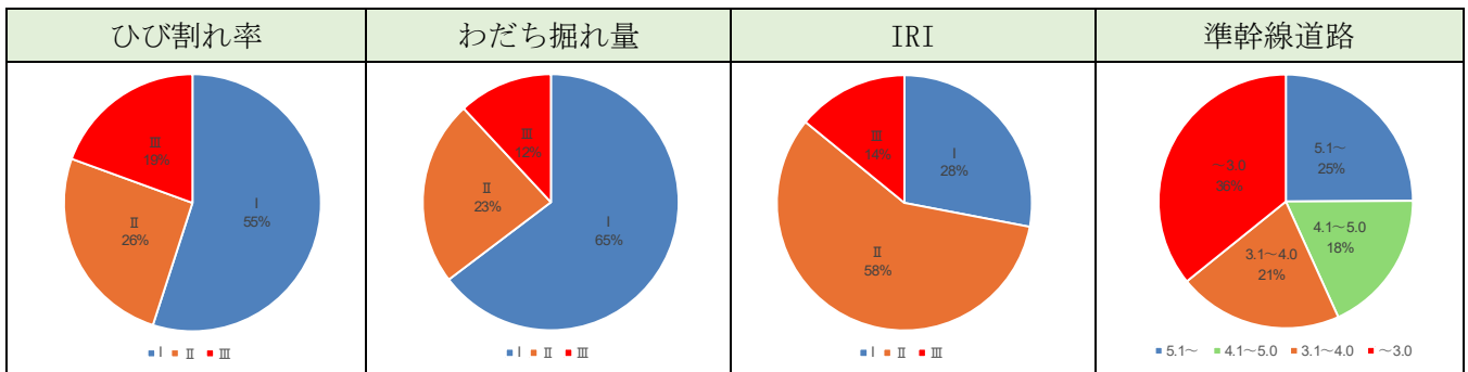
図 2-4 準幹線道路の診断区分割合比較
