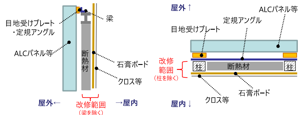
図2-3 横から見た断面図
