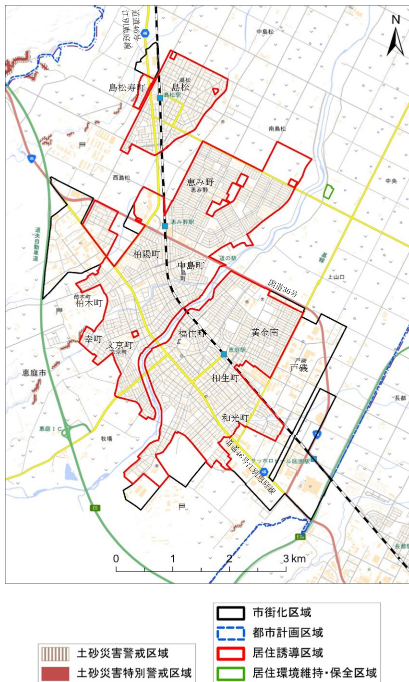
図 9.4 土砂災害警戒区域・土砂災害特別警戒区域
