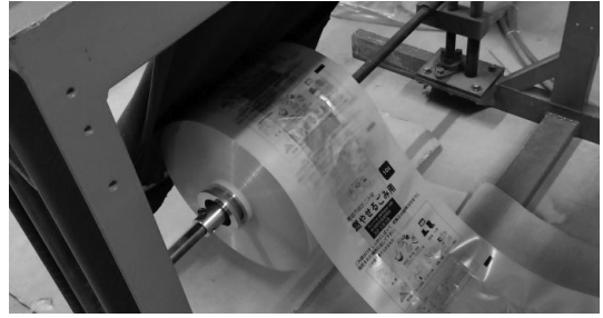
工場から届いたロールを製袋機にセット
