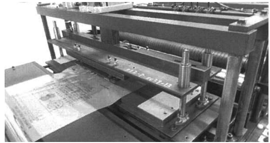
機械により熱溶着してカット
