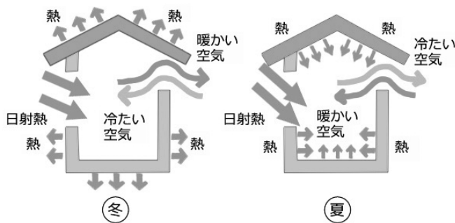
住宅の内外での熱の移動
